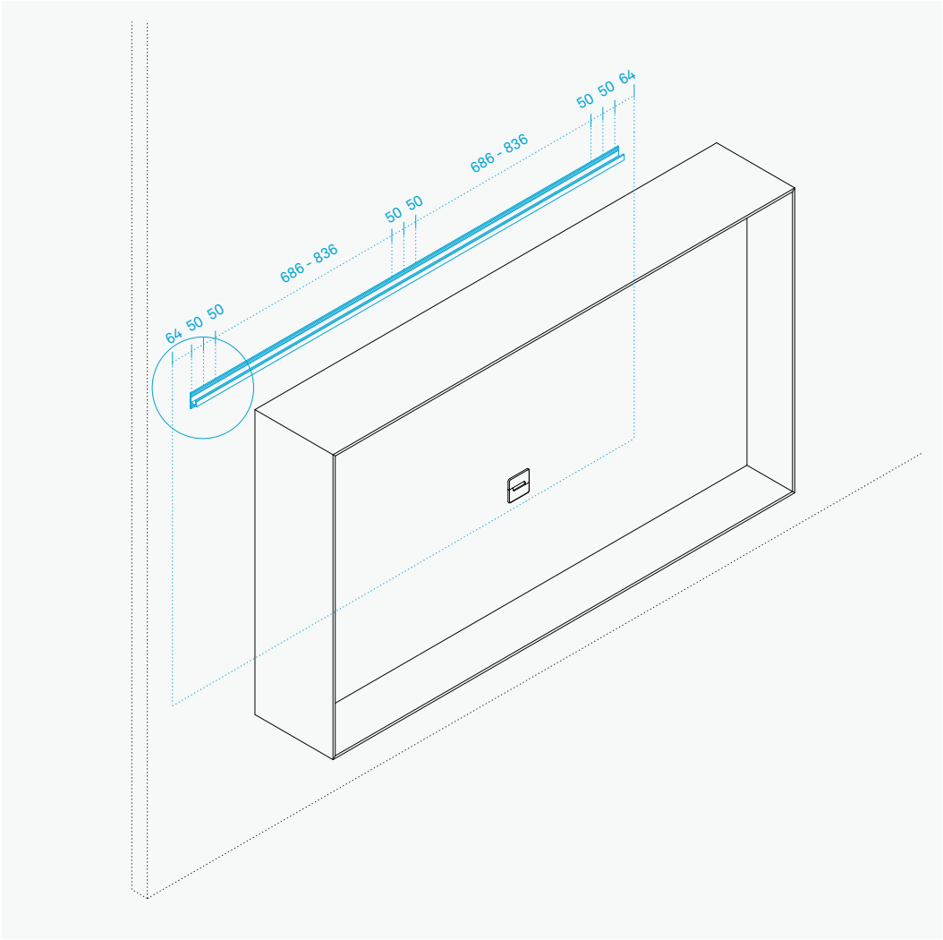
Barra per fissaggio in dotazione. Barre de fixation fournie.
