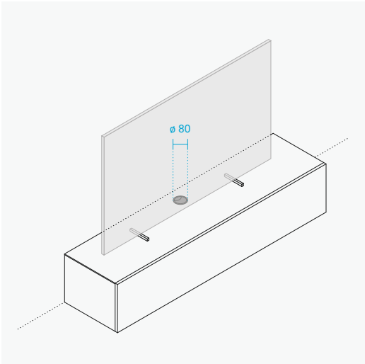
TV in appoggio con passacavo Titanio Brunito. TV en appui avec passe-câble Titanio Brunito.
