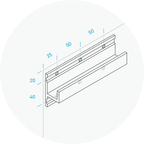
Per larghezza 300 ÷ 350. Pour largeur 300 ÷ 350.
