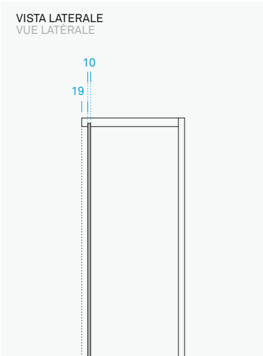
Spazio tecnico e schiena. Espace technique et dos.
