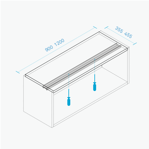
Barra di sostegno Titanio Brunito con possibilità di regolazione. Barre de support Titanio Brunito avec possibilité de réglage.
