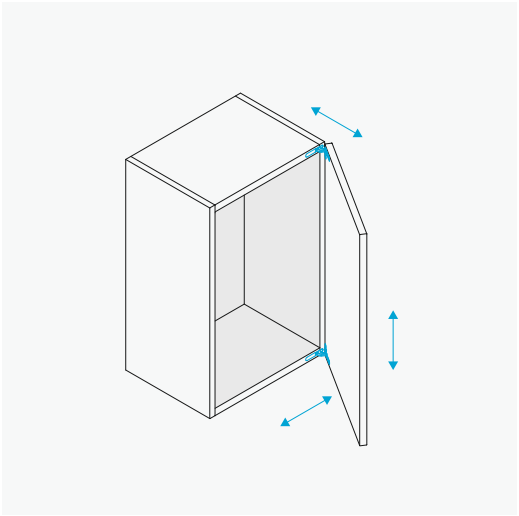
Tre regolazioni possibili. Trois réglages possibles.
