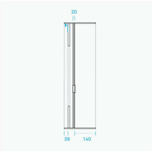
Spazio tecnico e schiena. Espace technique et dos.
