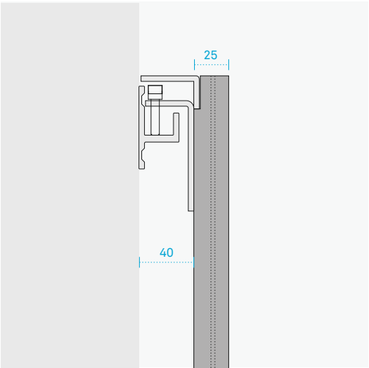
Spazio tecnico Espace technique
