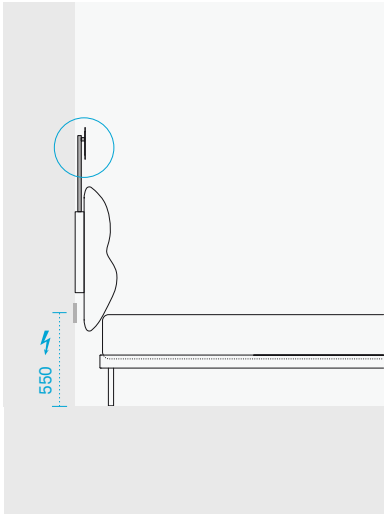
Alimentazione elettrica tramite presa a parete. Alimentation électrique par prise murale.
