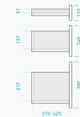
VISTA LATERALE VUE LATÉRALE
