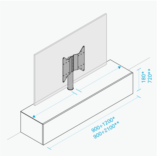
Posizionamento sempre al centro. Positionnement toujours au centre.
