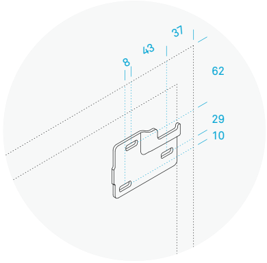
1. Staffa in dotazione. Support fourni.
