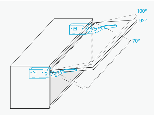
Ribalta superiore Abattant supérieur
