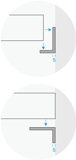
Profilo di sostegno Titanio Brunito. Due modalità di fissaggio a parete. Profil de support Titanio Brunito. Deux modes de fixation au mur.
