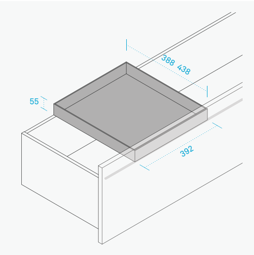
Vassoio Easy Pelle per cassetto H 360, larghezza 1050 e 1200. Plateau Easy Cuir pour tiroir H 360, largeur 1050 et 1200.
