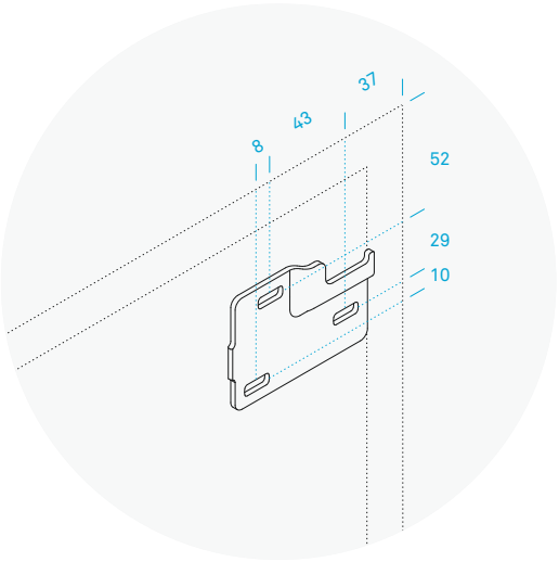
Staffa in dotazione. Support fourni.
