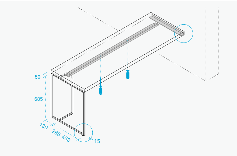
Barra di sostegno Titanio Brunito con possibilità di regolazione per L 1500 e 1800. Barre de support Titanio Brunito avec possibilité de réglage pour L 1500 et 1800.
