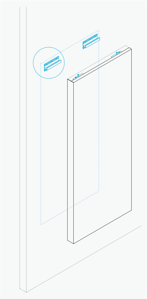
Barre per fissaggio in dotazione. Barres de fixation fournies.
