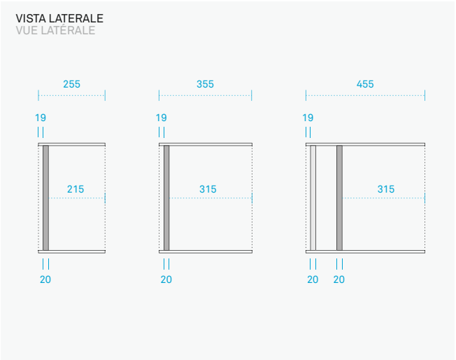
Spazio tecnico e schiena. Espace technique et dos.
